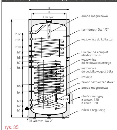
schemat wymiennika SGW(S)M Tower Multi 300-500
