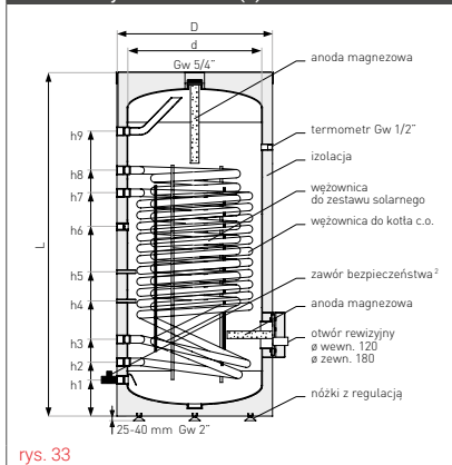
schemat wymiennika SGW(S)B Tower Biwal Max 200
