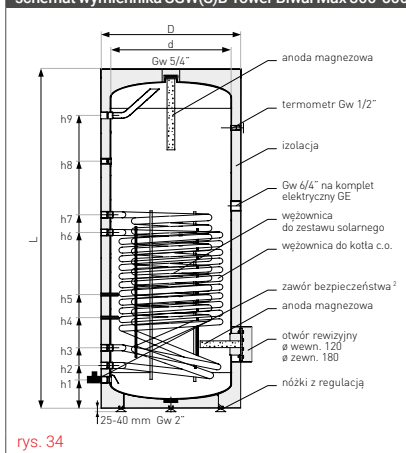
schemat wymiennika SGW(S)B Tower Biwal Max 300-500
