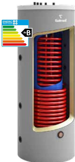
foto 28 SG(K) Kumulo z dwiema wężownicami
