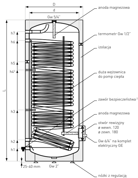
schemat wymiennika SGW(S) Tower Grand
